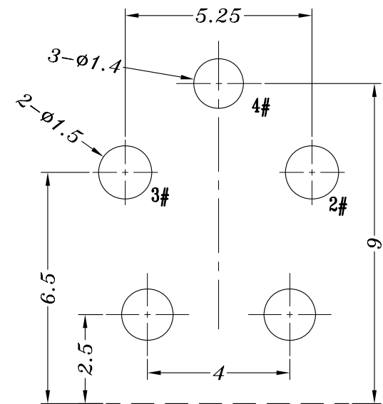
P.C.B LAYOUT
