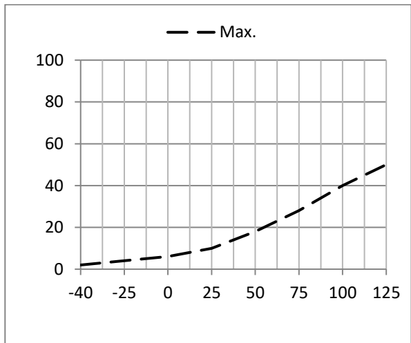
图 11B 悬浮电源漏电流 vs 温度
