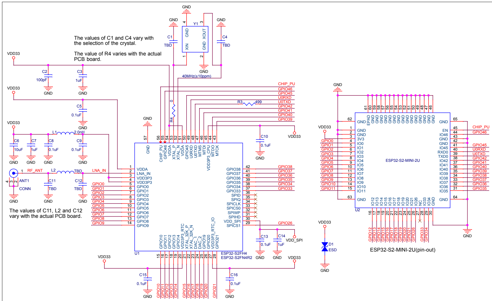
图 6: ESP32-S2-MINI-2U 原理图
