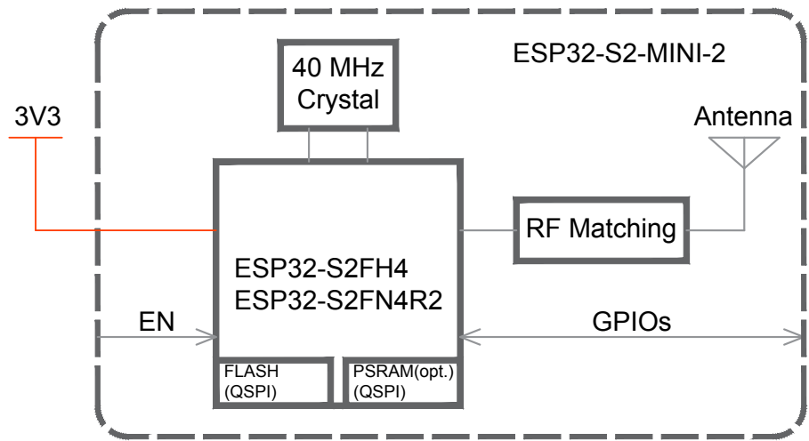
图 1: ESP32-S2-MINI-2 功能框图
