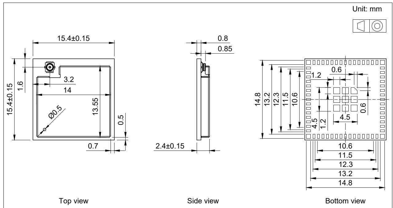
图 9: ESP32-S2-MINI-2U 模组尺寸
