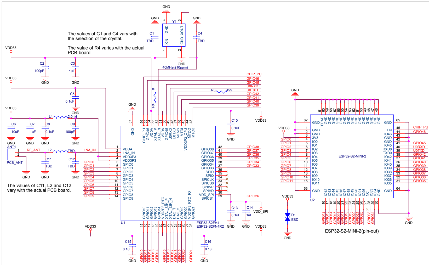
图 5: ESP32-S2-MINI-2 原理图
