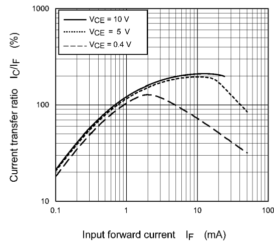
Fig. 11.12 I_C/I_F - I_F
