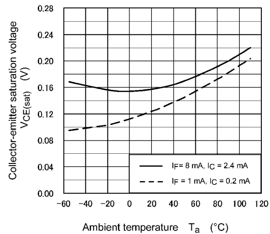
Fig. 11.10 V_{CE(\text{sat})} - T_a
