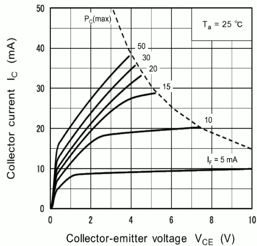
Fig. 11.7 I_C - V_{CE0}
