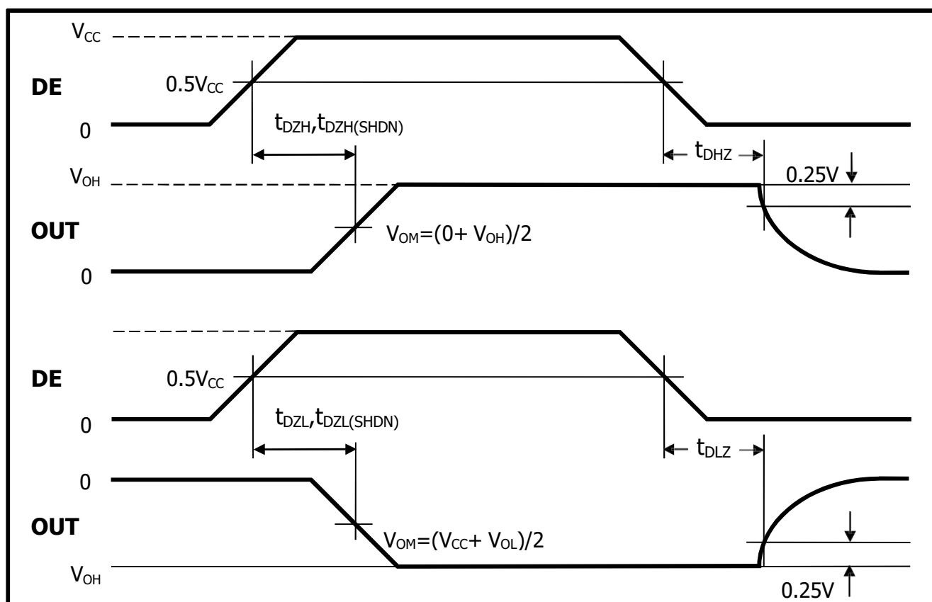
图 6.驱动器使能和禁用时序( t_{DZH} 、 t_{DZL} 、 t_{DZH}(SHDN) 、 t_{DZL} 、 t_{DLZ} 、 t_{DLZ}(SHDN) )
