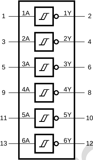
图 1 逻辑符号
