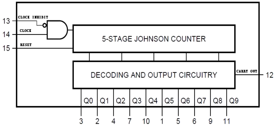
图 1 功能框图
