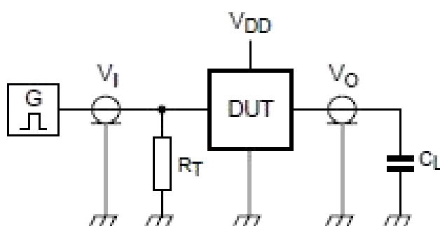
图 9 测试电路
