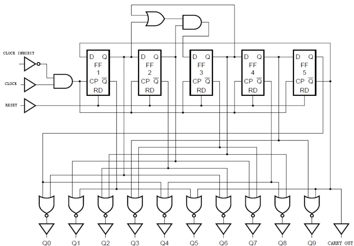
图 3 逻辑图
