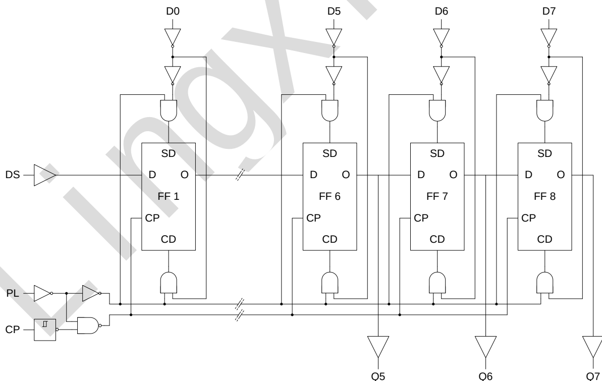
图 2. 逻辑图
