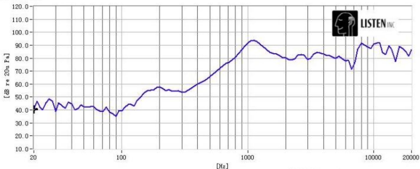
頻响曲线
