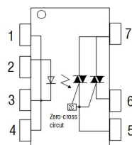
Zero-on 过零型
