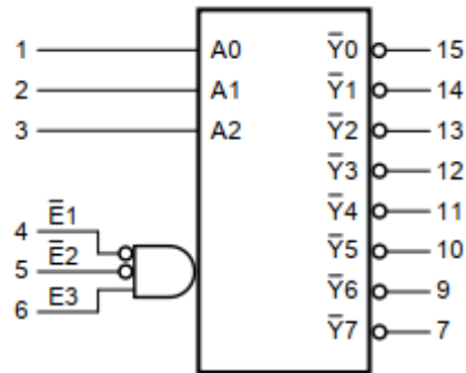
图 1 逻辑符号
