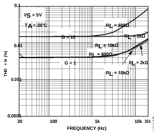
图38. 总谐波失真加噪声与频率的关系
