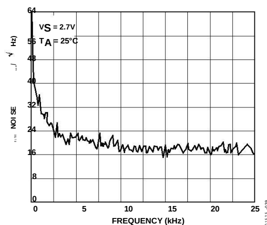
图39. 电压噪声密度与频率的关系
