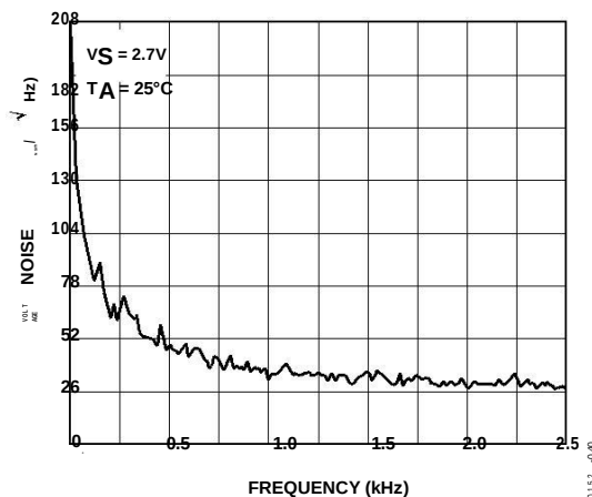
图40. 电压噪声密度与频率的关系
