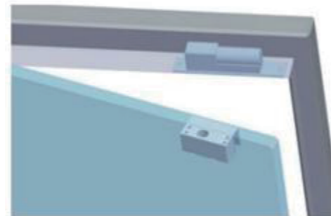
下无框玻璃门安装图
