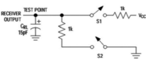
图4接收时间测试电路
