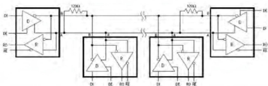
图 12 典型双工 RS-485 网络
