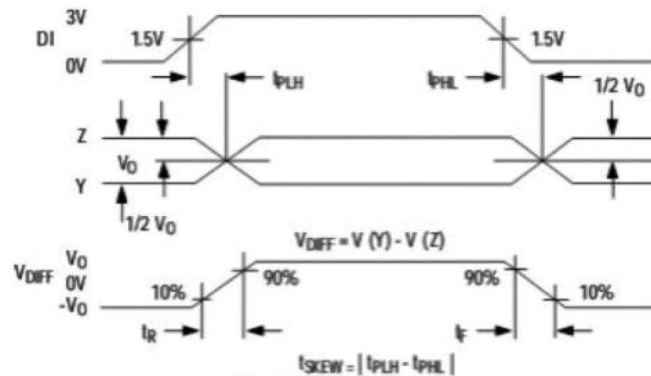
图 8 驱动传输延时
