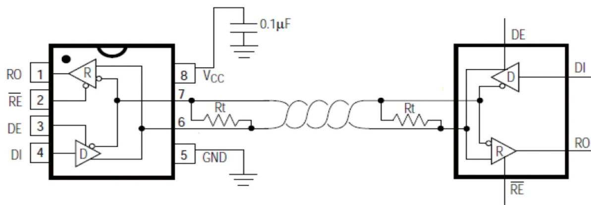
图1： SP3485ECN典型半双工应用电路
