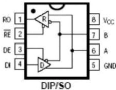
图1封装图
