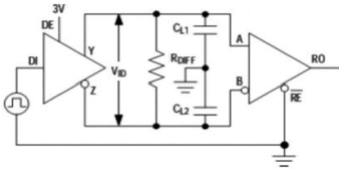
图6驱动时间测试电路
