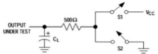
图6驱动时间测试电路
