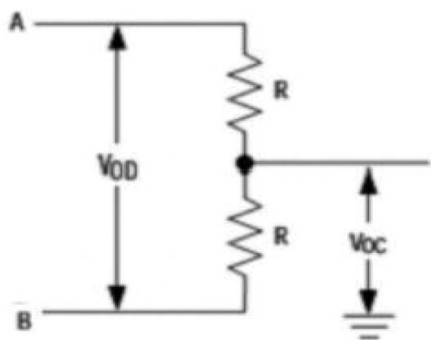
图3直流驱动测试电路
