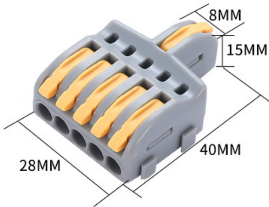
一进五出黄色接线端子
