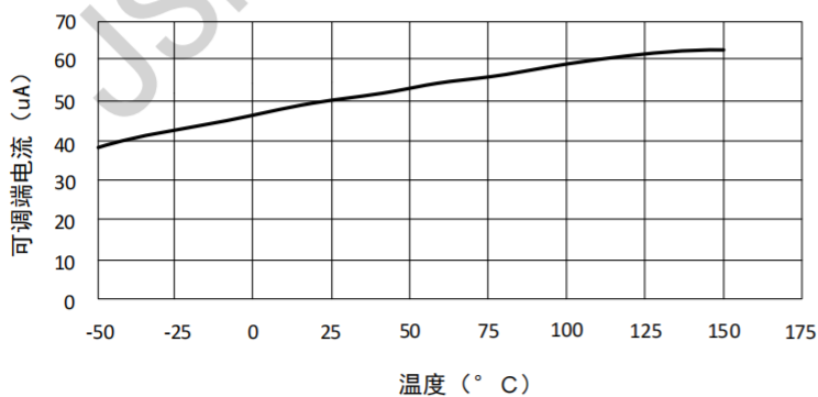
图 7 可调端输出电流随温度变化曲线
