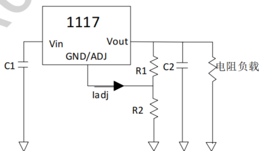
AMS1117CD可调版本典型应用图
