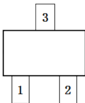
SOT-89 封装
