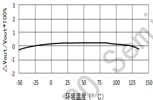
图 6 温度稳定性曲线
