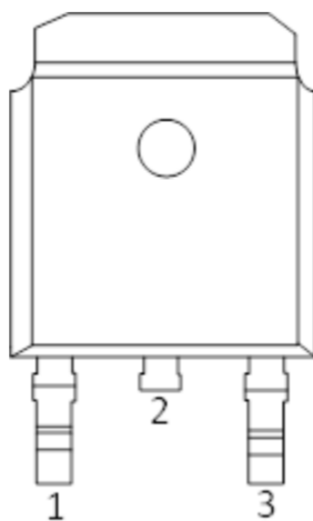
TO-252 封装
