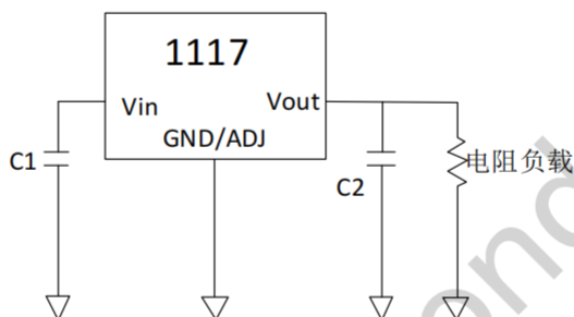
AMS1117CD固定电压版本典型应用图
