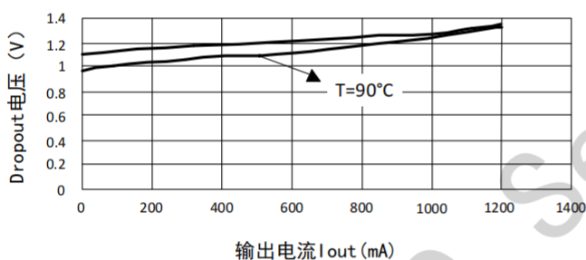
图1 不同负载时输入输出电压特性曲线
