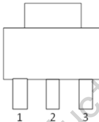
SOT-223 封装
