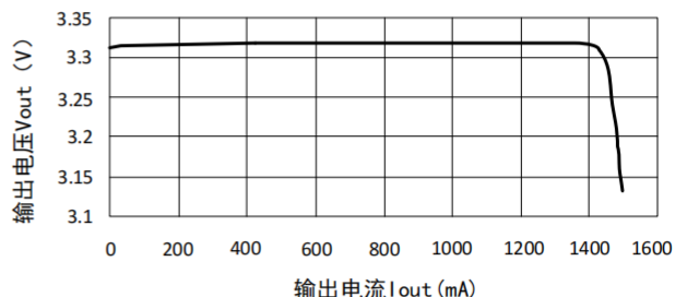
图4 负载特性曲线
