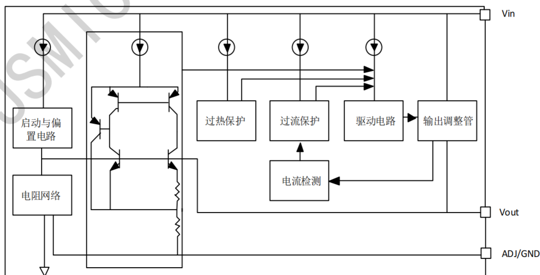
图1 AMS1117CD的内部结构图
