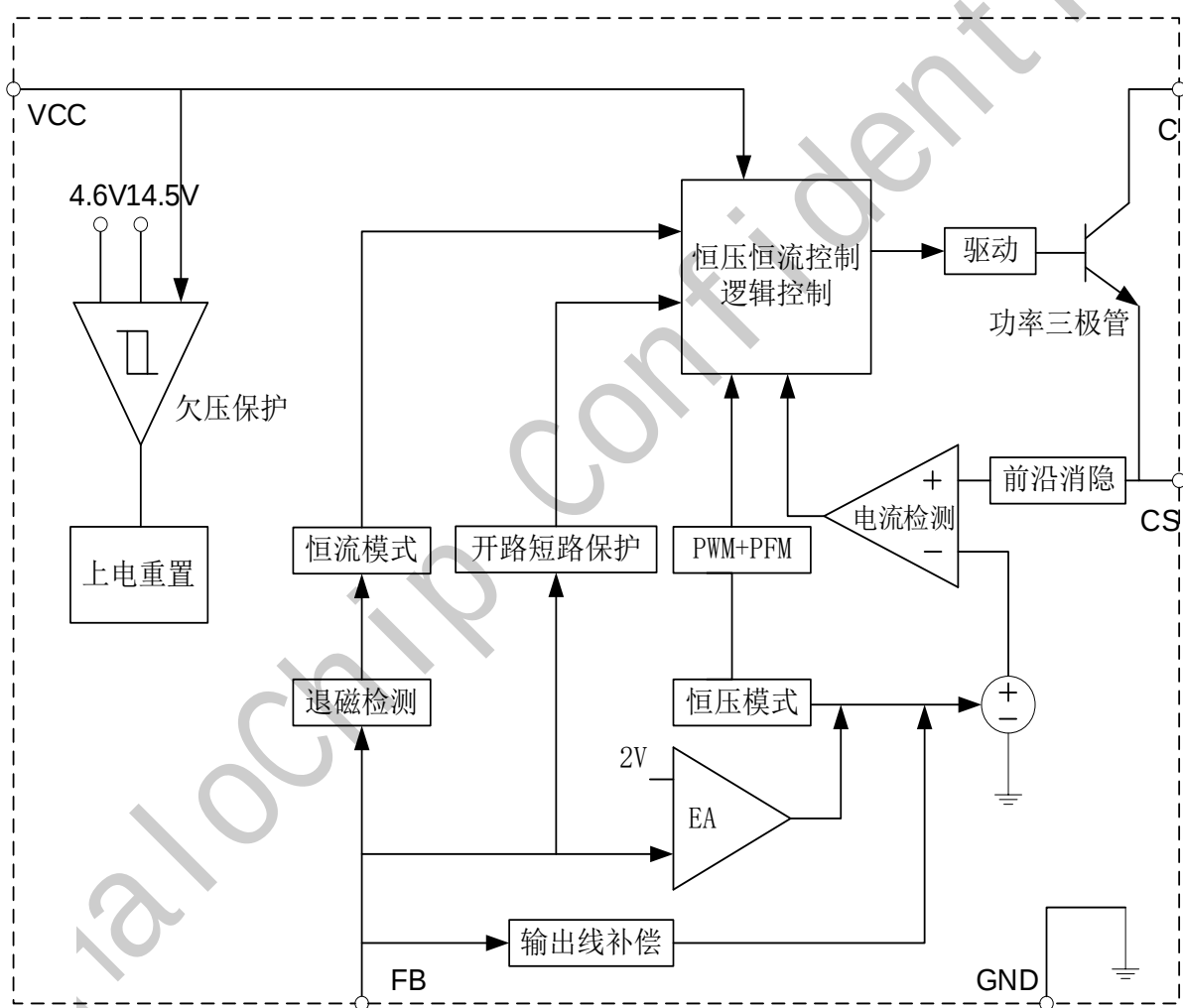
图 3 GP8631SE 内部框图
