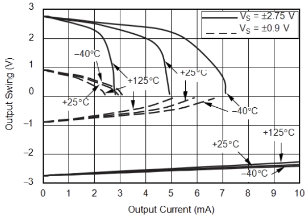
Figure 5. 输出电压摆幅与输出电流间的关系
