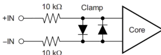
Figure 20. 等效输入电路
