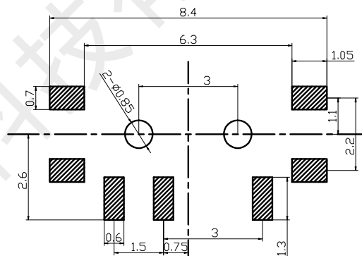
安装参考图
