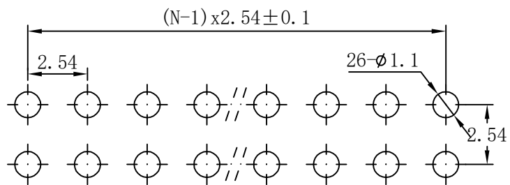
P.C.B Layout
