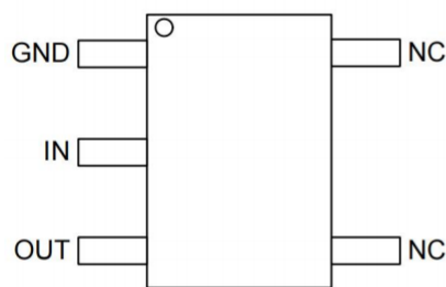
SOT23-5
