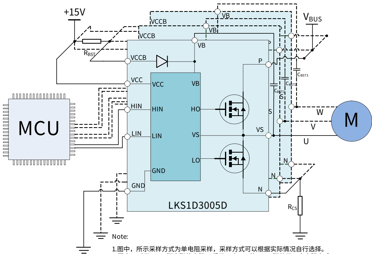
图 1. LKS1D3005D 典型应用图
