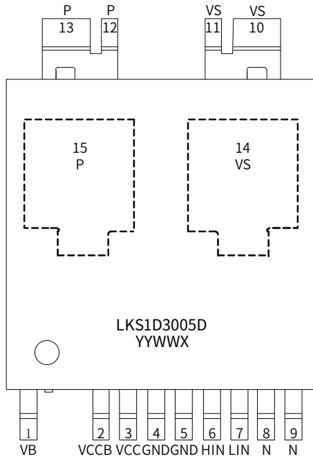
图 2. LKS1D3005D 管脚封装图
