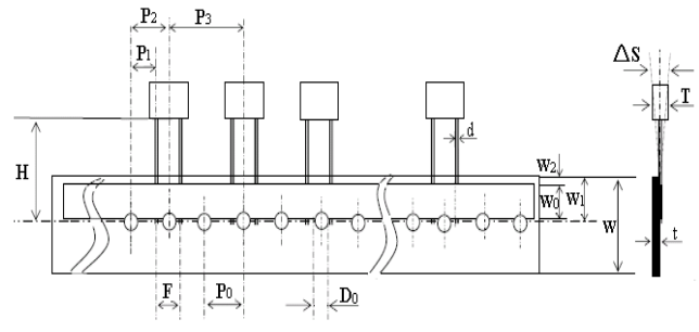
Fig.2 P=10.0, 15.0mm
