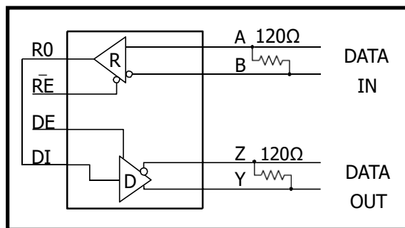
图 11. HGX3070E/ HGX3073E/ HGX3076E 全双工模式下的中继器
