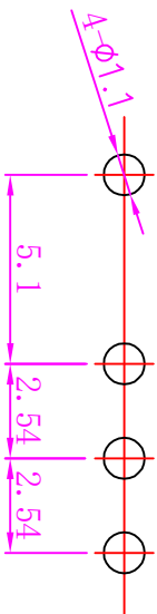
安装尺寸
