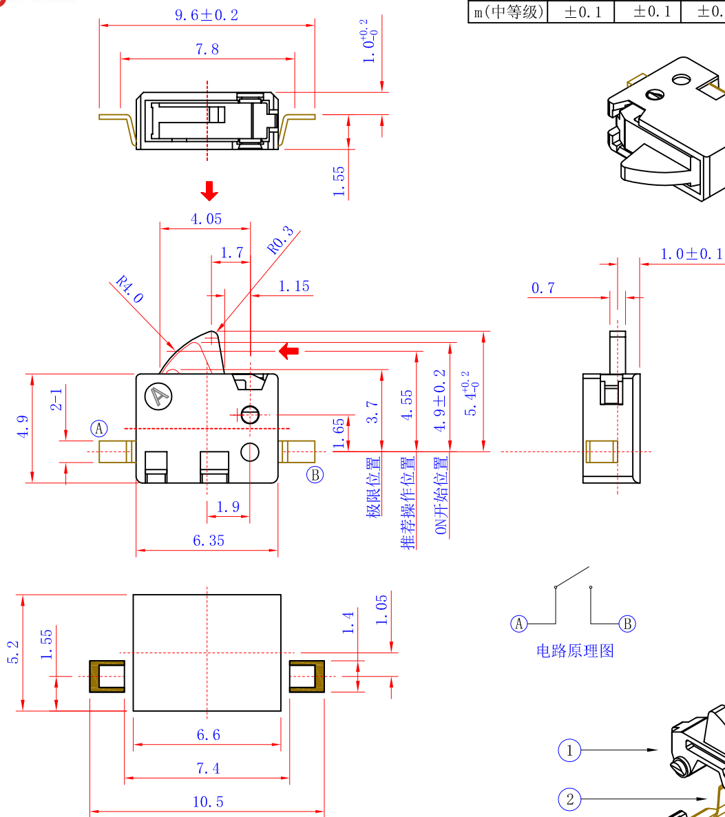
安装尺寸图
