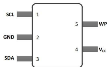
SOT-23-5
