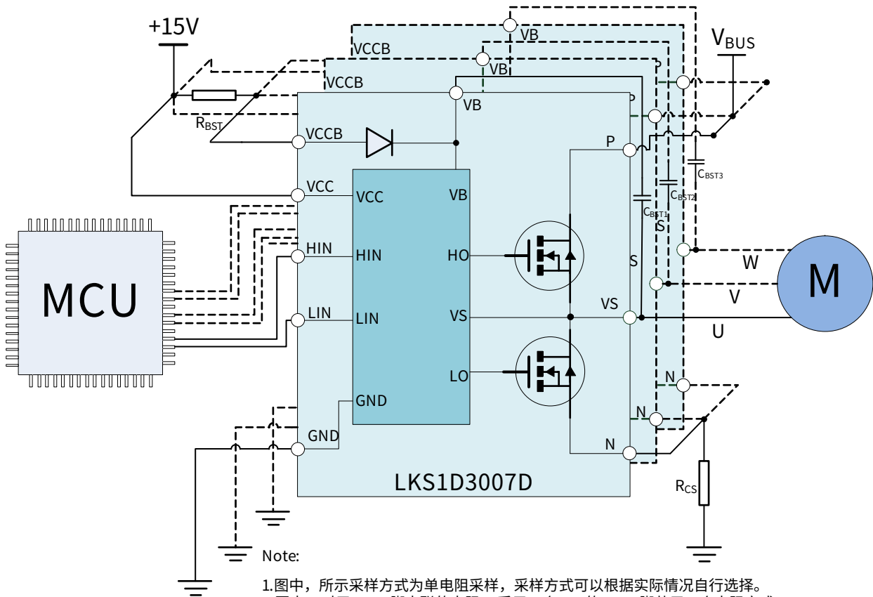
图 1. LKS1D3007D 典型应用图
