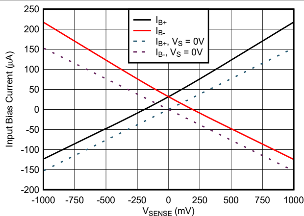
图 7-19. INA241x2-Q1 输入偏置电流与 V_{\text{SENSE}} 间的关系
