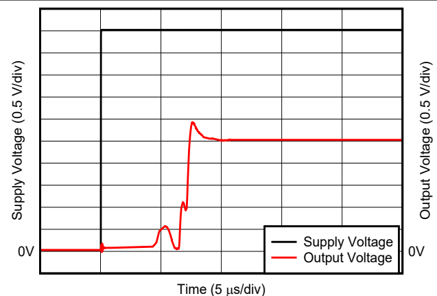
图 7-34. 小阶跃响应
