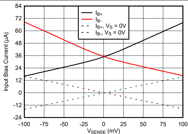
图 7-21. INA241x5-Q1 输入偏置电流与 V_{\text{SENSE}} 间的关系
