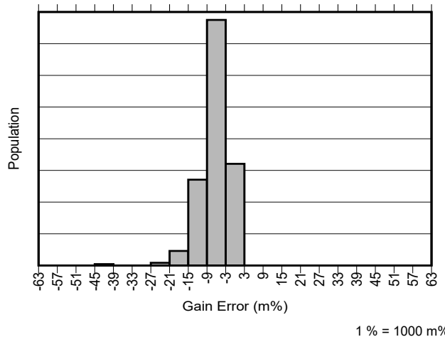
图 7-12. 所有增益 INA241B-Q1 增益误差产生分布图
