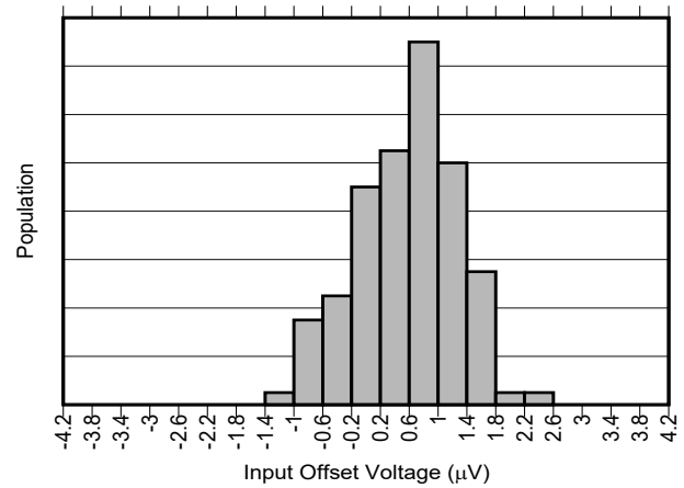
图 7-4. INA241A5-Q1 输入失调电压产生分布图
