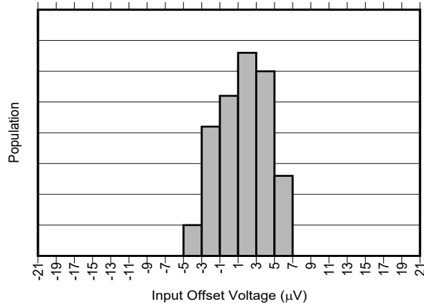
图 7-1. INA241A1-Q1 输入失调电压产生分布图
