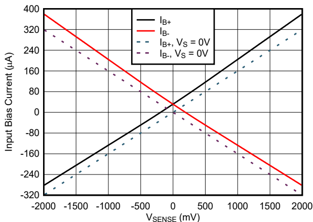
图 7-18. INA241x1-Q1 输入偏置电流与 V_{\text{SENSE}} 间的关系
