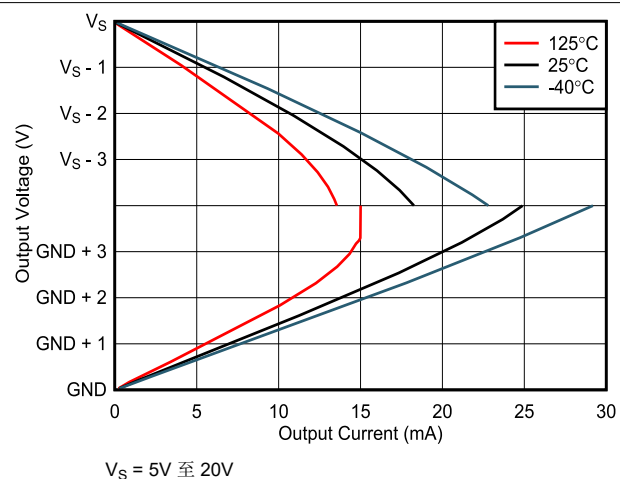
图 7-23. 输出电压与输出电流间的关系
