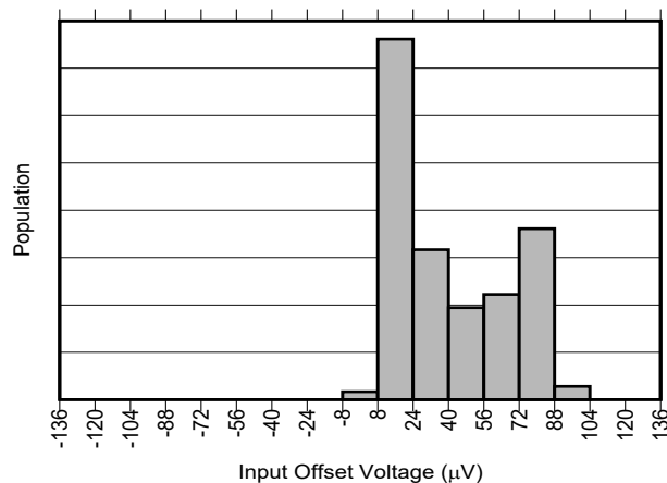
图 7-3. INA241A3-Q1 和 INA241A4-Q1 输入失调电压产生分布图
