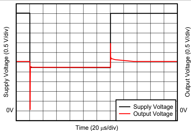
图 7-37. 欠压恢复
