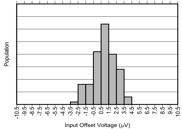
图 7-2. INA241A2-Q1 输入失调电压产生分布图
