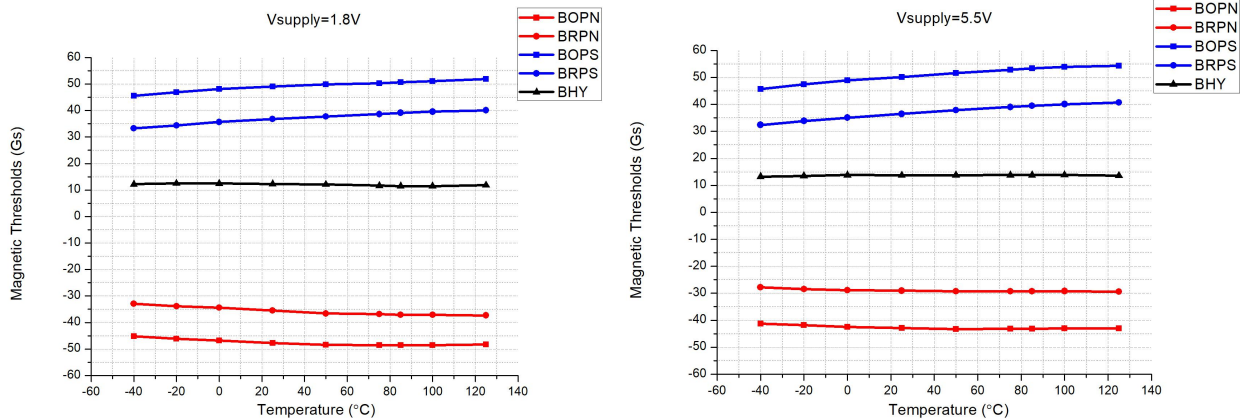
磁场阈值 vs 温度 @VDD=1.8V
