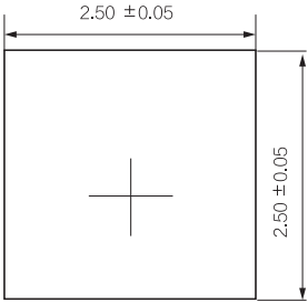
俯视图
