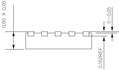
侧视图
