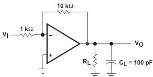
图 2. 10 倍增益电路
