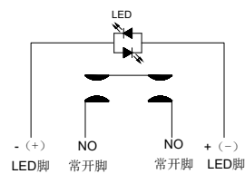
Schematic Diagram 电气原理图
