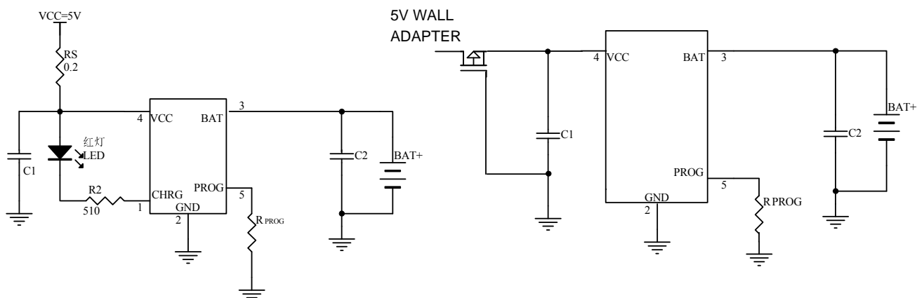
全功能单节锂电池充电器（接耗电电阻） （无电池状态红灯闪烁）
