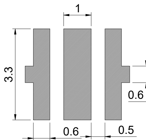
焊盘建议图
