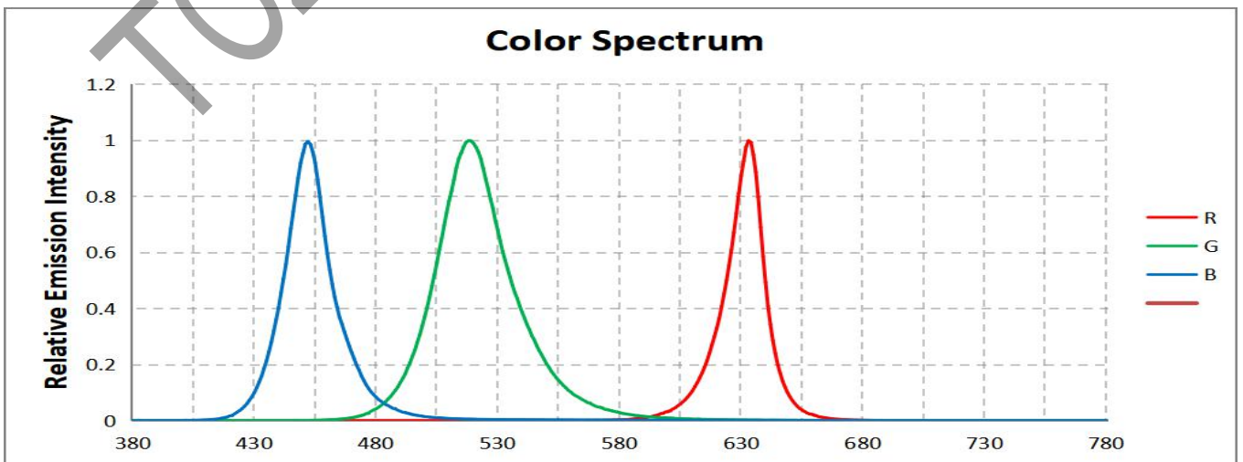
光谱图, Ta=25°C
