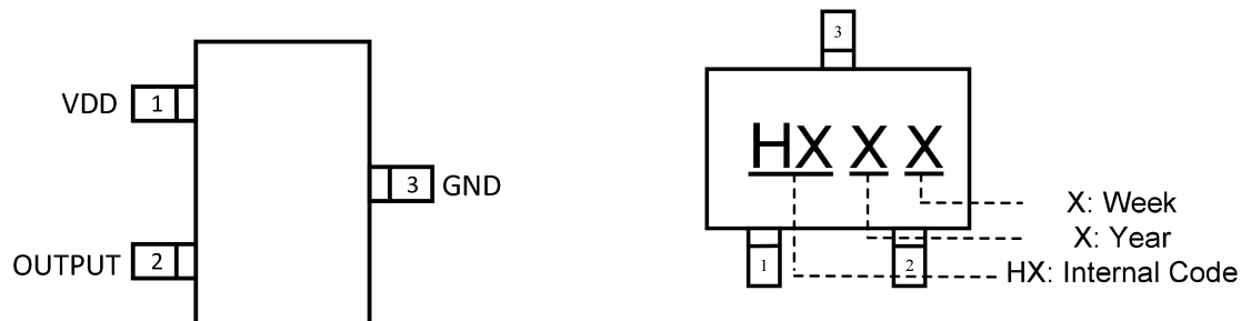
SOT-23-3L
