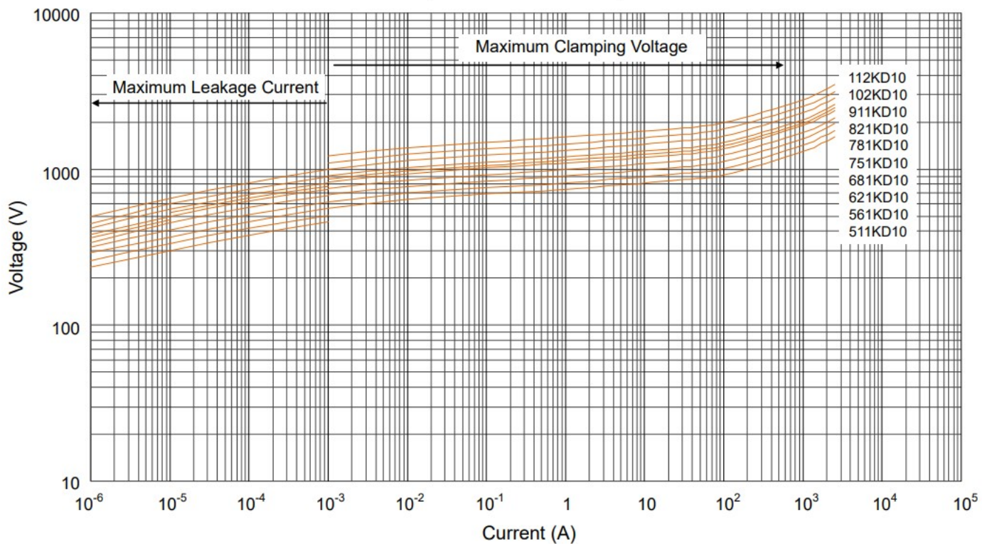
511KD10 to 112KD10
