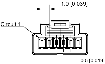
端面 X1004H-XXA-NOHF
