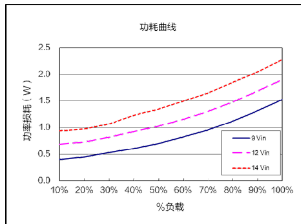
功耗曲线 ( V_{out}=5.4V )
