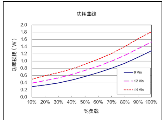
功耗曲线 ( V_{out}=1.2V )
