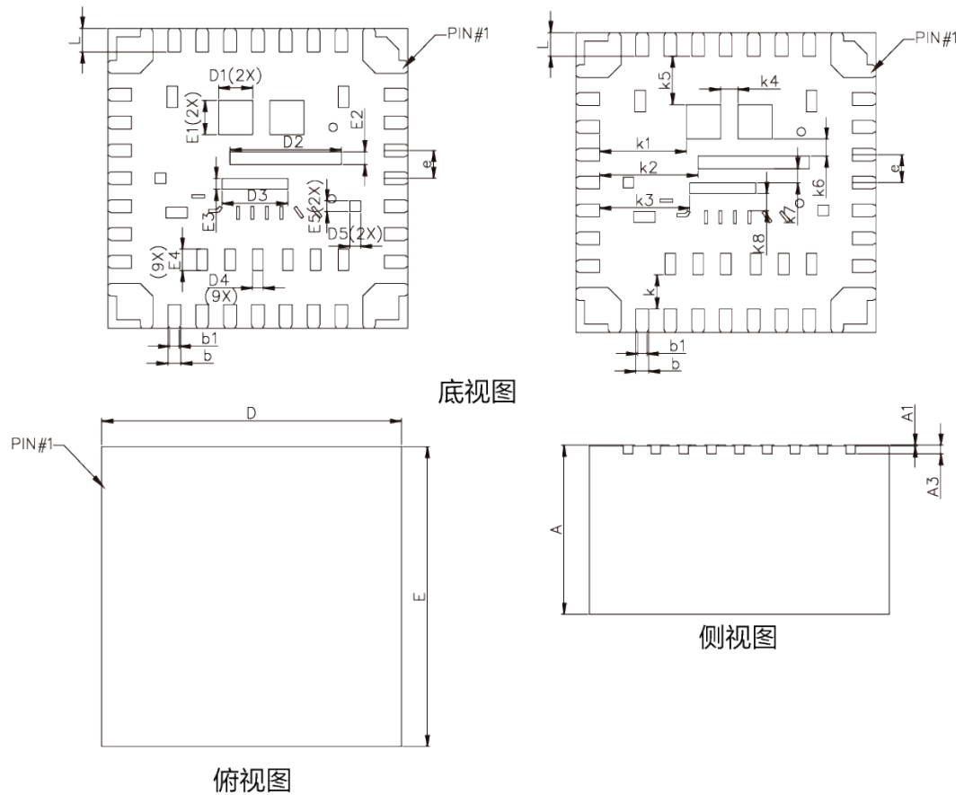
图 6-2 结构尺寸图
