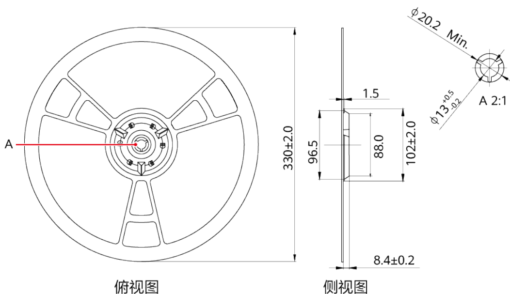
图 12-1 卷盘尺寸
