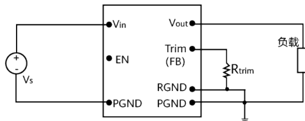
图 6-5 R trim 外部连接
