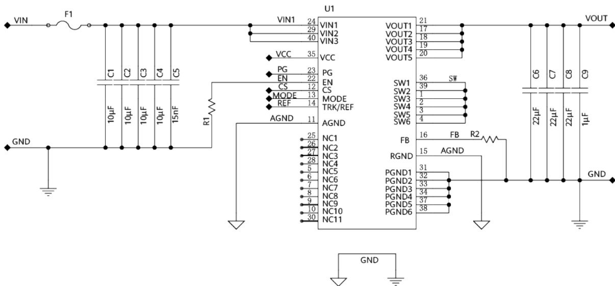
图 5-1 推荐应用电路
