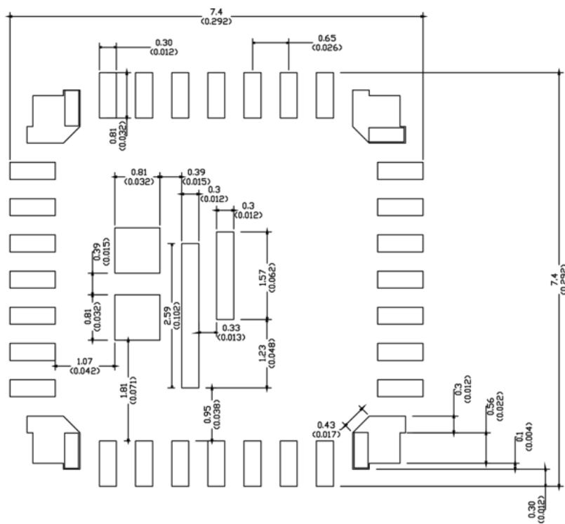
图 6-1 封装尺寸图
