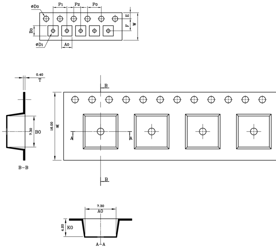
图 12-2 卷带尺寸
