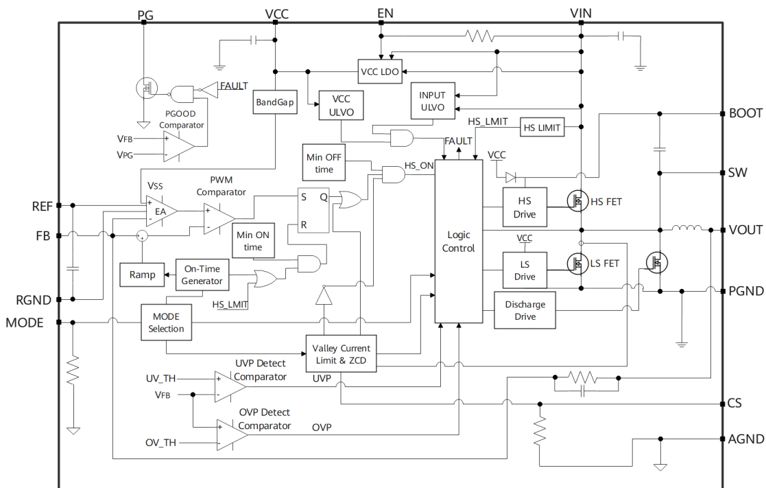
图 3-1 原理框图
