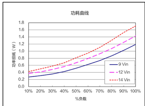
功耗曲线 ( V_{out}=0.7V )
