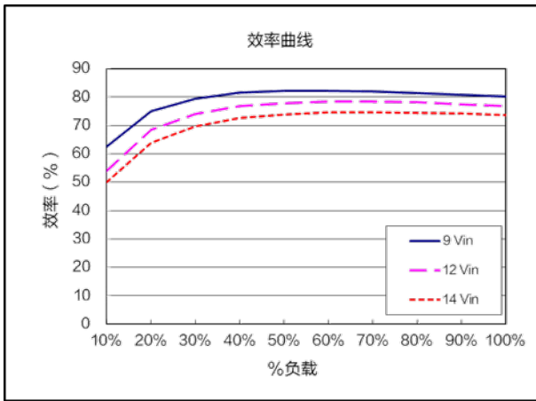
效率曲线 ( V_{out}=0.8V )
