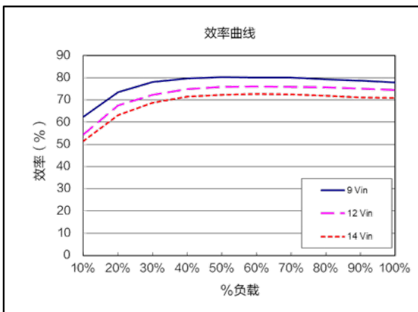
效率曲线 ( V_{out}=0.7V )
