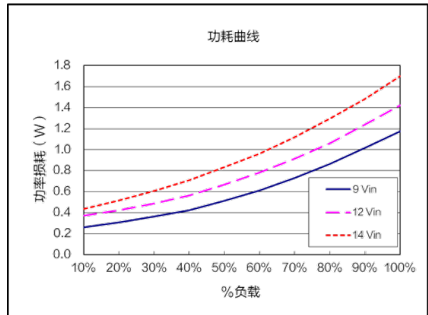
功耗曲线 ( V_{out}=0.8V )
