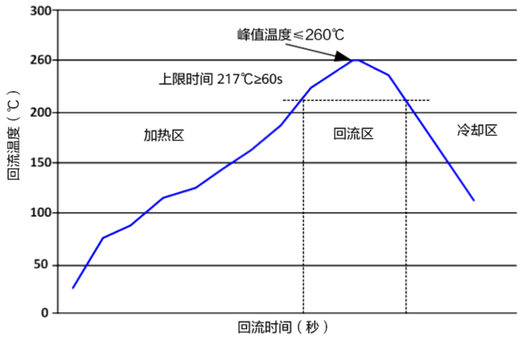
图 10-2 推荐无铅焊接回流曲线
