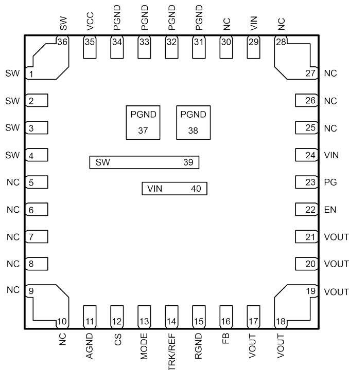
图 6-3 引脚分布
