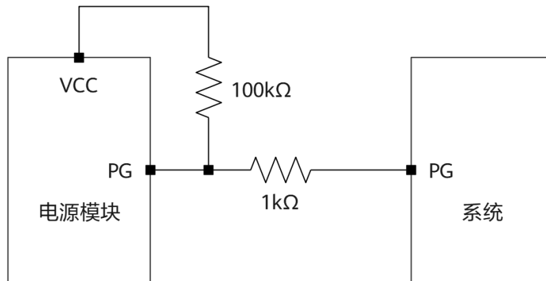
图 6-6 PG 信号配置图
