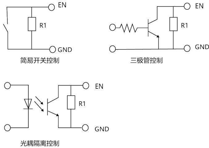
图 6-4 EN 引脚控制方式推荐图
