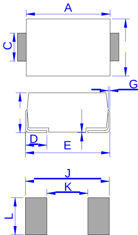
DO-214AC (SMA)
