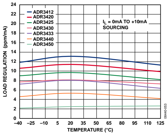
图5. 负载调整率与温度的关系(源电流)
