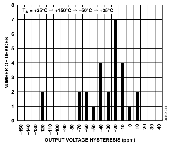
图37. ADR3450热致输出电压迟滞分布图
