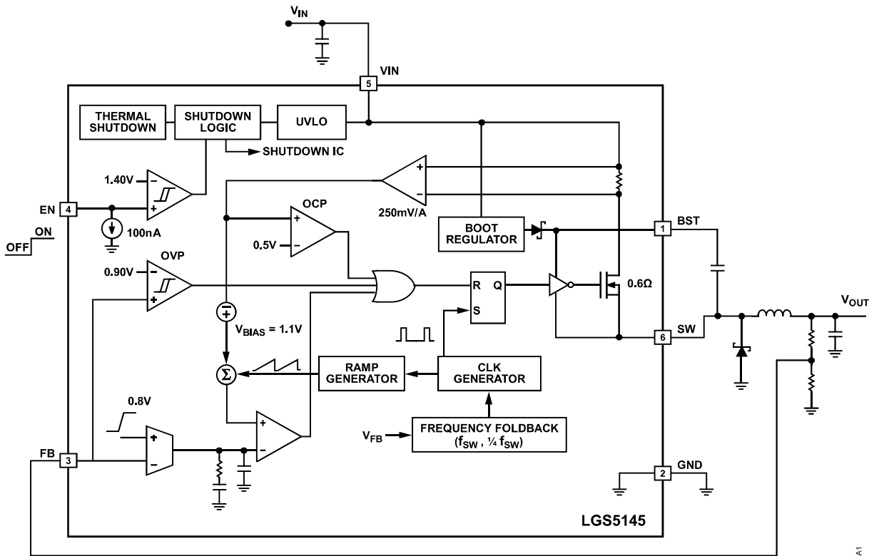
图4 内部框图
