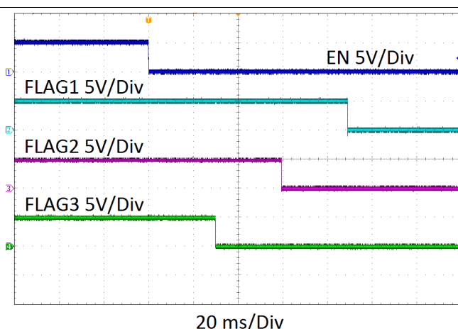
图 17. LM3880MF-1AE 的下电序列
