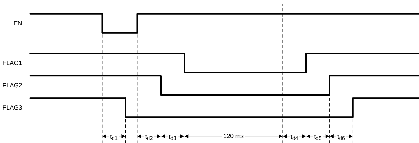
图 14. 不完整的下电序列
