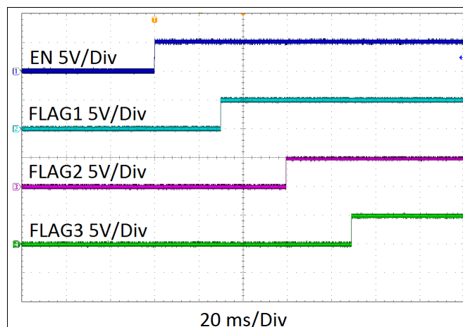
图 16. LM3880MF-1AE 的上电序列
