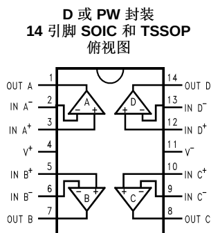
引脚功能
