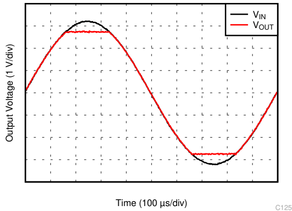
图 6-25. No Phase Reversal
