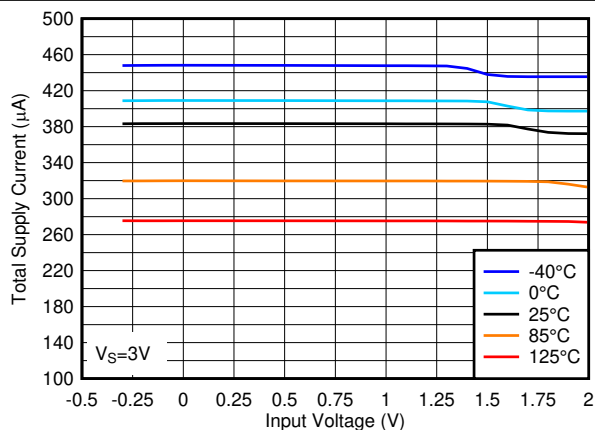
图 6-7. 3V 下总电源电流与输入电压之间的关系
