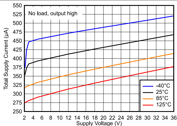
图 6-6. 总电源电流与电源电压之间的关系
