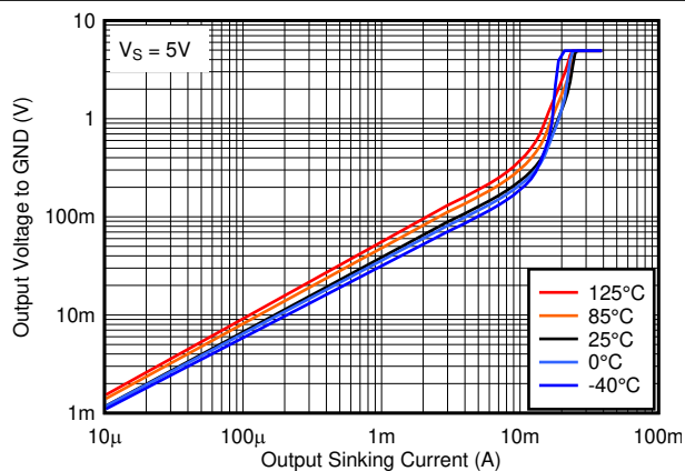
图 6-25. 5V 下输出低电平电压与输出灌电流之间的关系
