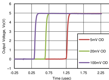
图 8-2. 各种过驱的响应时间 (正转换)
