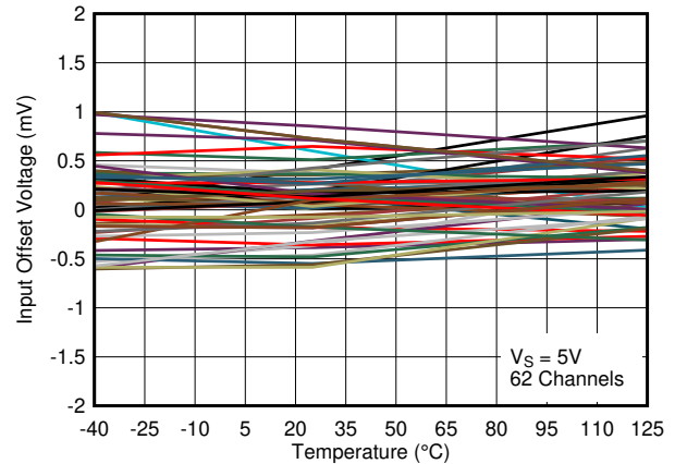
图 6-13. 5V 下输入失调电压与温度之间的关系
