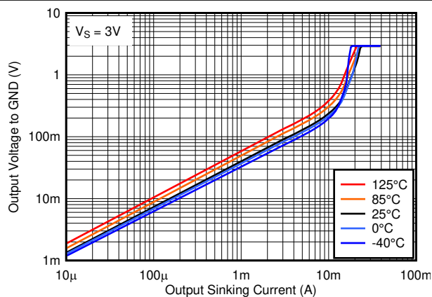
图 6-24. 3V 下输出低电平电压与输出灌电流之间的关系
