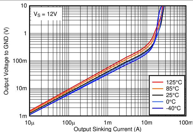
图 6-26. 12V 下输出低电平电压与输出灌电流之间的关系
