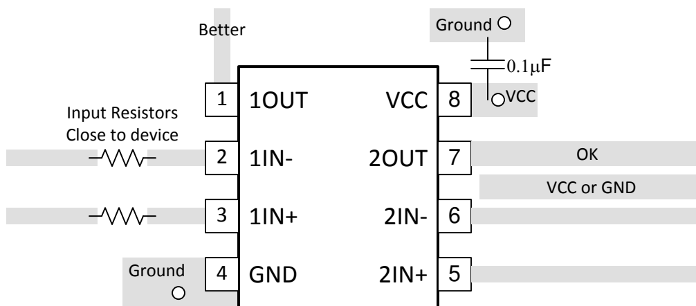
图 10-1. LM2903 布局示例
