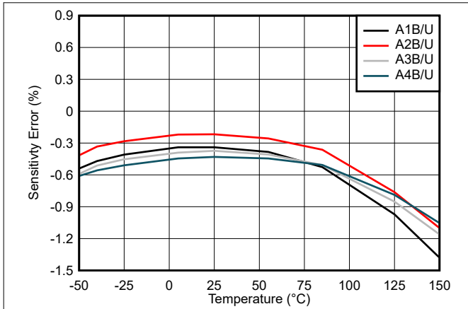
图 7-1. TMCS1107 灵敏度误差与温度间的关系
